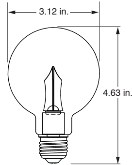
Globe 25 E26 Base
