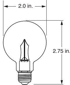
Globe 16.5 E26 Base
